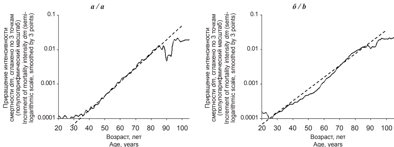
Рис. 3. Изменения скорости старения для России во второй половине XX в: a – 1960 г.; b – 1980 г.
