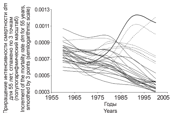
Рис. 2. Изменения скорости старения для 30 стран во второй половине XX в.
